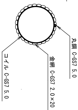
断面図
